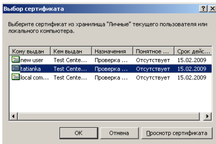
Рис. 36. Выбор сертификата
