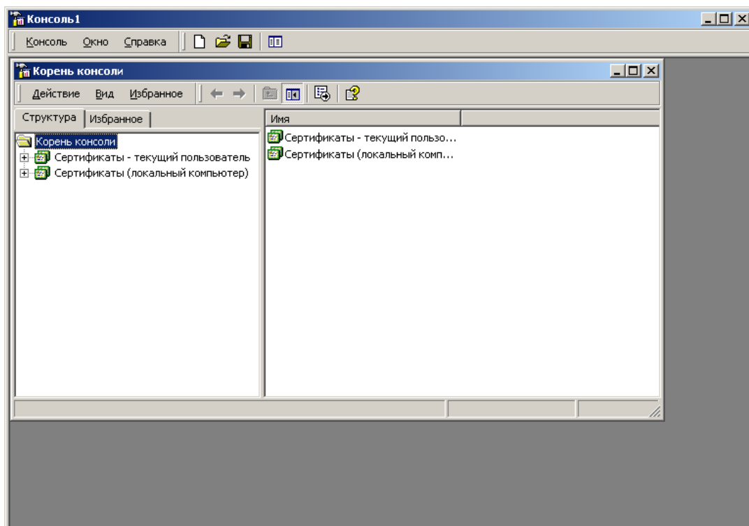
Рис. 79. Консоль MMC
